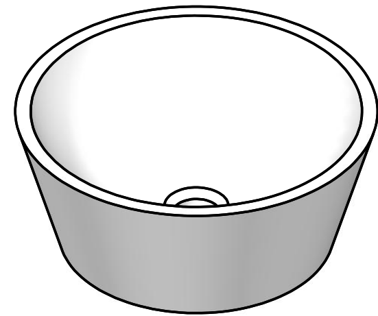
Aufsatzbecken D601 Außen d=350mm h=145mm ohne Überlauf
