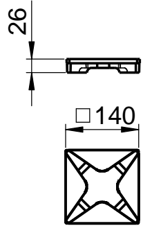
Detail Ablauf
