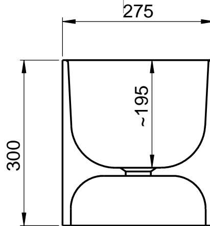
A-A (1:7)
